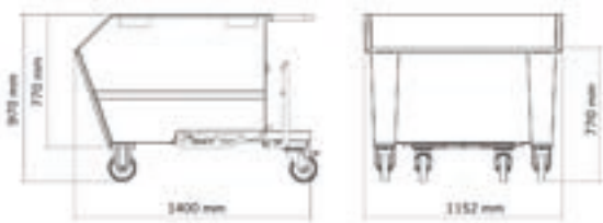
Benna portarottami ribaltabile capacità 750 L con ruote predisposta per griglia e rubinetto
